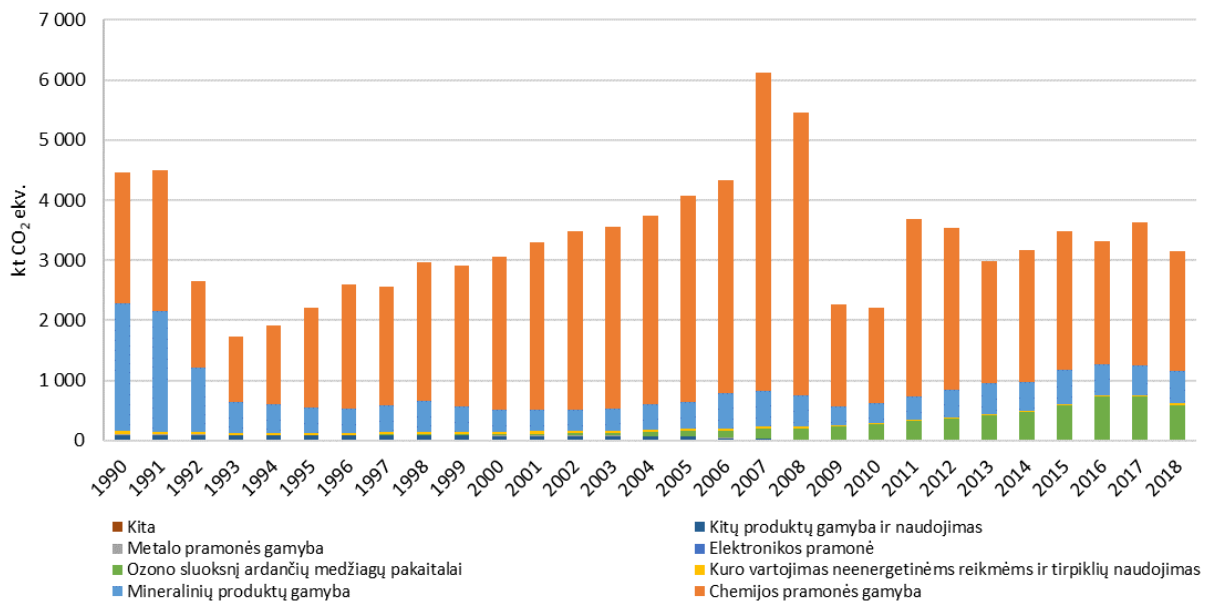
7 pav. Išmetamų ŠESD kiekio tendencijos pramonės procesų ir pramonės produktų naudojimo sektoriuje Lietuvoje 1990-2018 m., kt CO 2 ekv.
