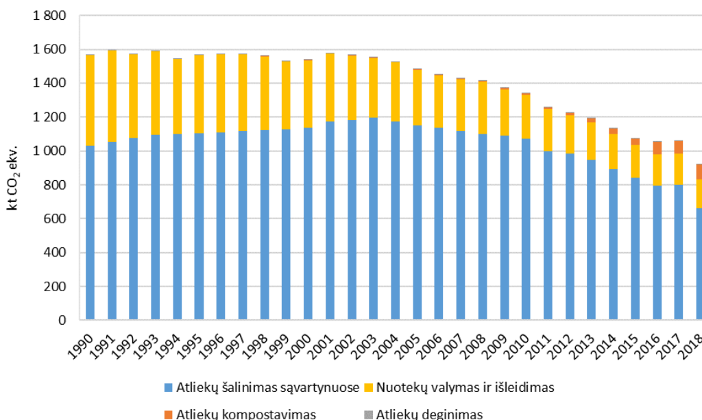
11 pav. Išmetamų ŠESD kiekio kitimas atliekų sektoriuje Lietuvoje 1990-2018 m. laikotarpiu, kt CO 2 ekv.
