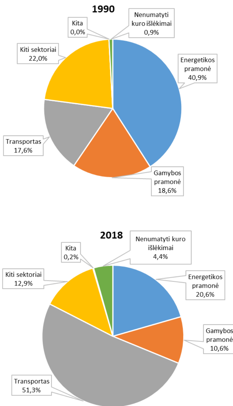
6 pav. Išmetamų ŠESD kiekis (%) energetikos sub-sektoriuose 1990 m. ir 2018 m.
