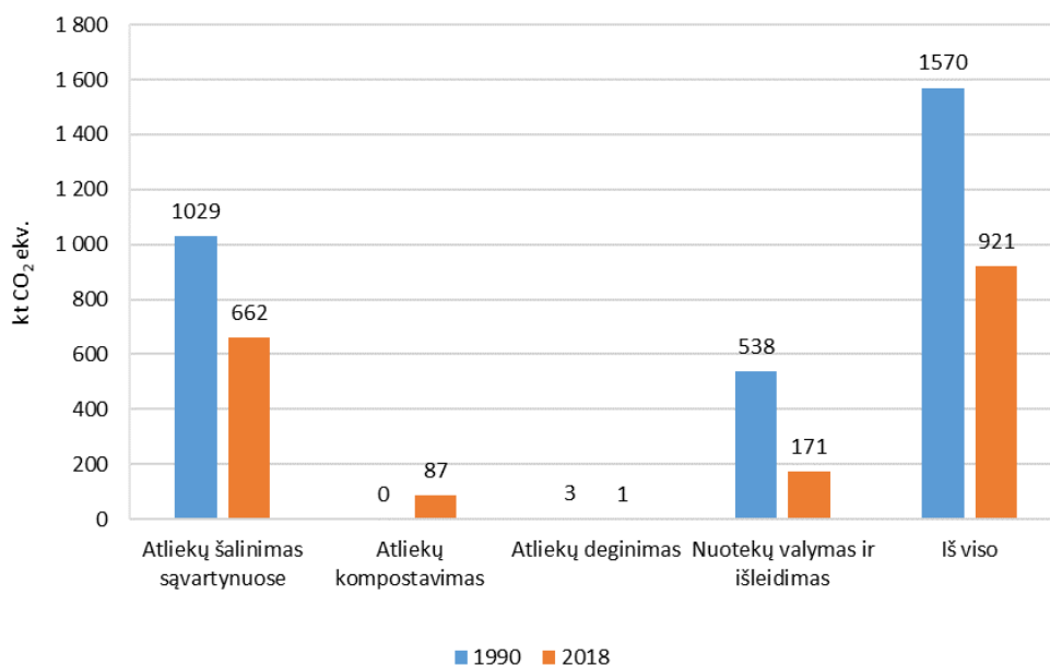
12 pav. Išmetamųjų ŠESD kiekio atliekų sektoriuje palyginimas tarp 1990 ir 2018, kt CO 2 ekv.
