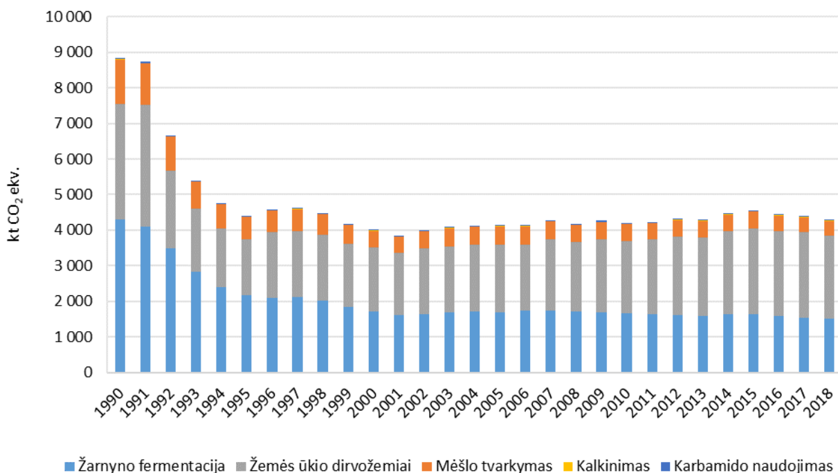
8 pav. Išmetamų ŠESD kiekio tendencijos žemės ūkio sektoriuje Lietuvoje 1990-2018 m., kt CO 2 ekv.
