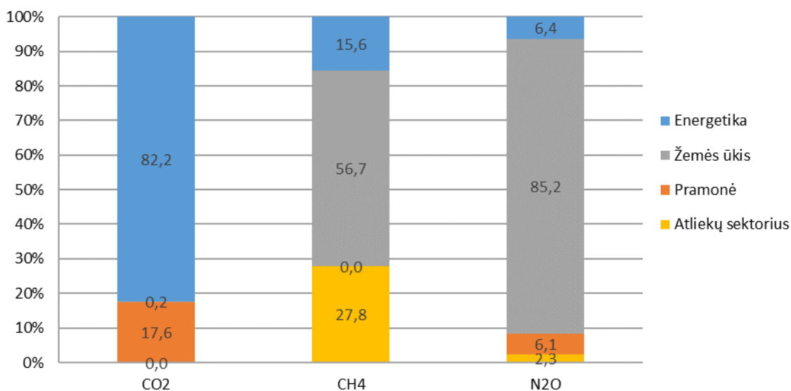
2 pav. Lietuvoje susidaręs ŠESD (CO 2 , CH 4 , N 2 O) kiekis (%) skirtinguose sektoriuose, 2018 m.
