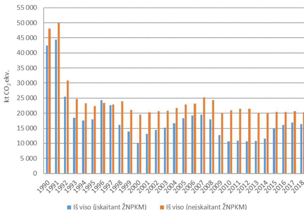
3 pav. Lietuvoje išmetamų ŠESD kiekio kitimo tendencija 1990-2018 m., kt CO 2 ekv.
