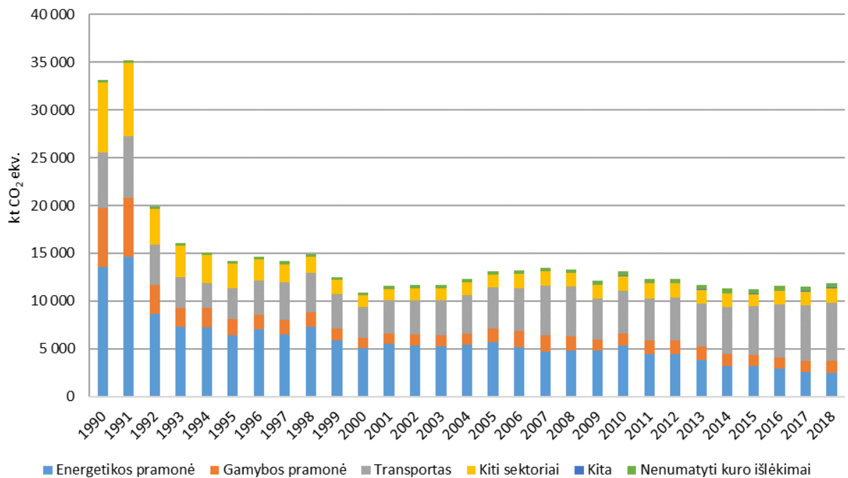
5 pav. Išmetamų ŠESD kiekio tendencijos energetikos sektoriuje Lietuvoje 1990-2018 m., kt CO 2 ekv.
