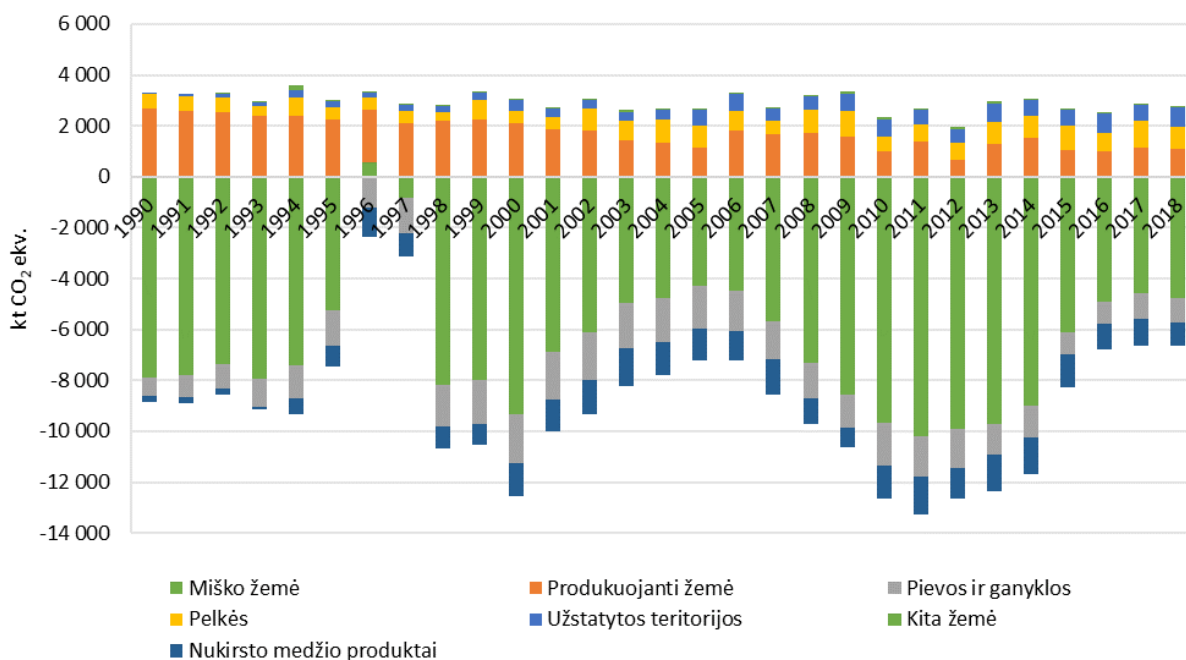
10 pav. Išmetamų ŠESD kiekio ir sugerties (absorbicijos) tendencijos žemės naudojimo, žemės naudojimo paskirties keitimo ir miškininkystės sektoriuje Lietuvoje 1990-2018 m., kt CO 2 ekv.
