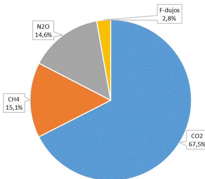
4 pav. Lietuvoje išmetamų ŠESD sudėtis 2018 m., CO 2 ekv. neįskaitant ŽNPKM
