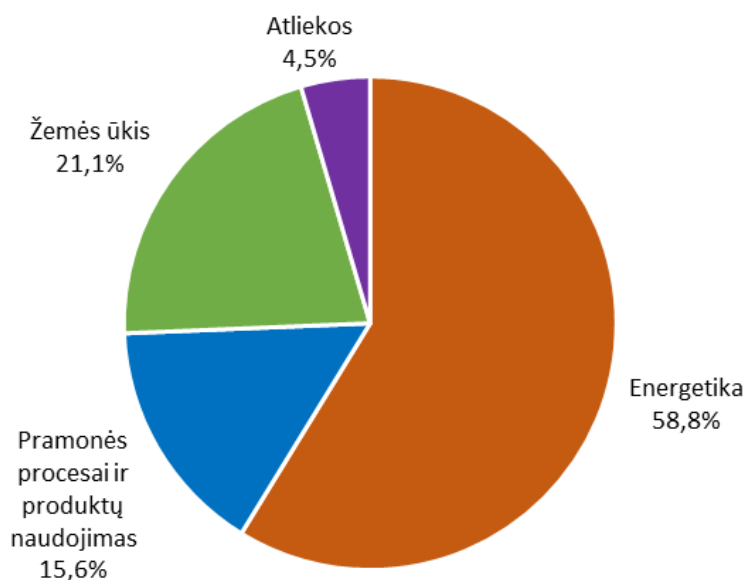
1 pav. Lietuvoje susidaręs ŠESD kiekis (%) pagal sektorius 2018 m.
