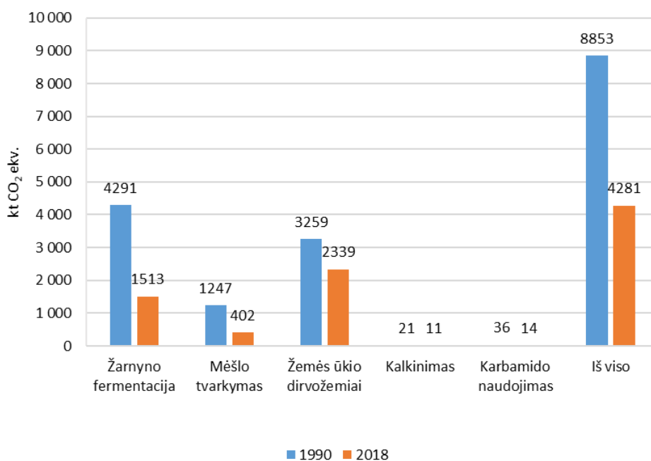
9 pav. Išmetamų ŠESD kiekio žemės ūkio sektoriuje palyginimas tarp 1990 ir 2018 m., kt CO 2 ekv.
